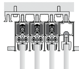
Trojkrídlový systém s fixným dielom namontovaný na nosný kompenzačný profil na strop.
