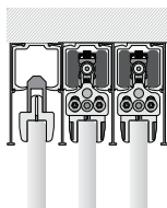
Dvojkridlový systém s fixným dielom s montážou na strop.
