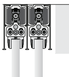
Dvojkridlový systém bez fixného dielu s montážou na strop vedľa steny.
